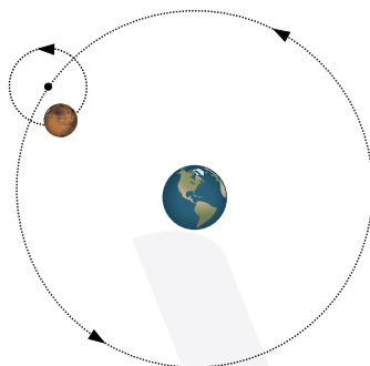
Geocentrična teorija
